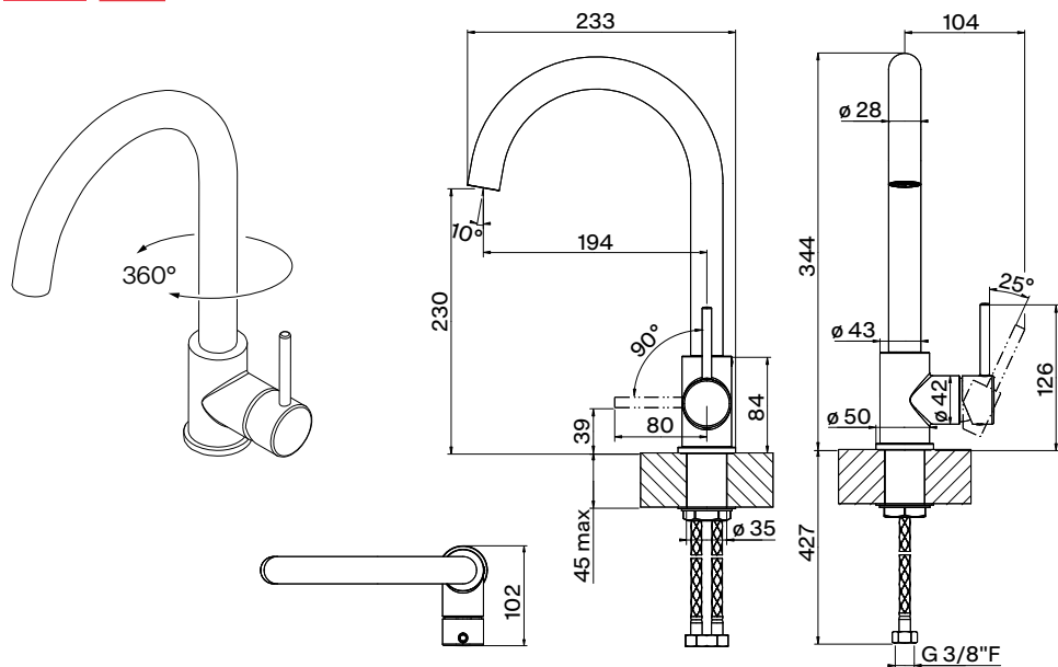
Tap Pola J Swivel side HP
