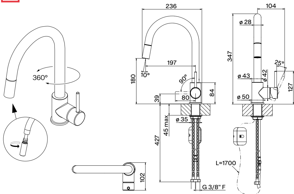
Tap Pola J Pull Down HP
