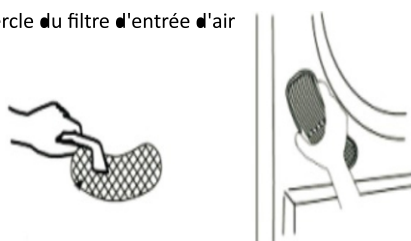
Couvercle du filtre d'entrée d'air
